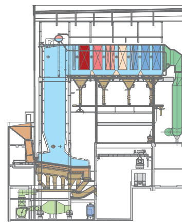
Exemple d'installation alimentée en ordures ménagères et déchets assimilés d'artisans
